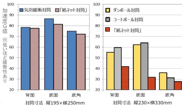
④各種封筒と「紙ネット封筒」の緩衝性比較
